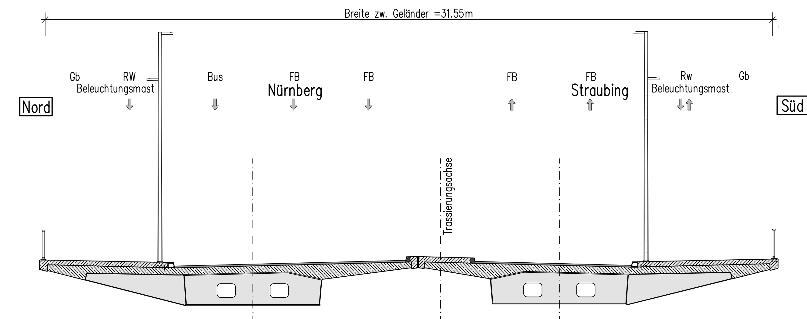
REGELQUERSCHNITT M 1:100 Brücke
