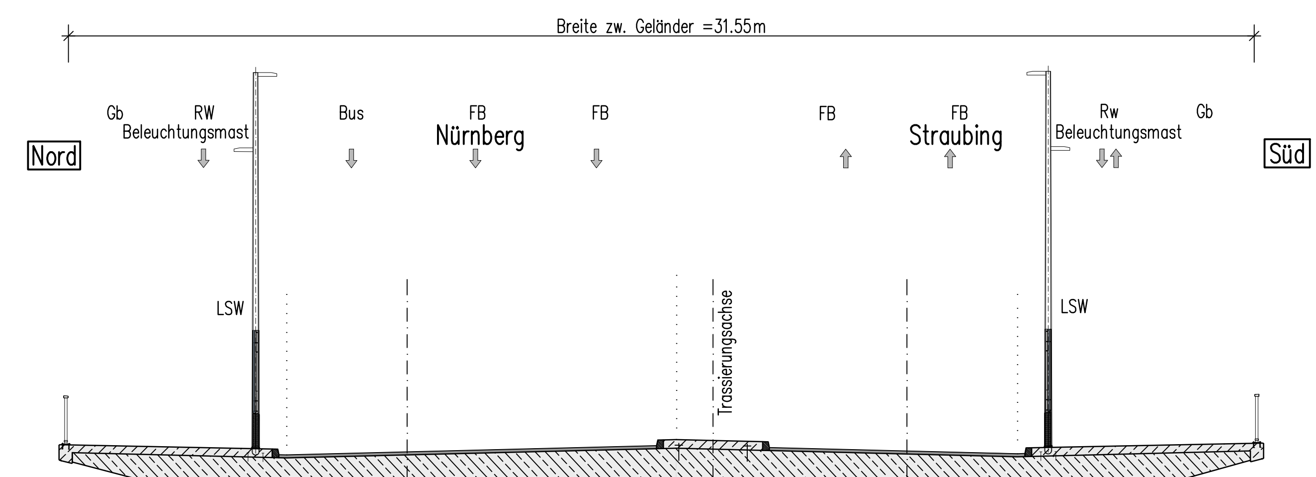
REGELQUERSCHNITT M 1:100 Rahmen
