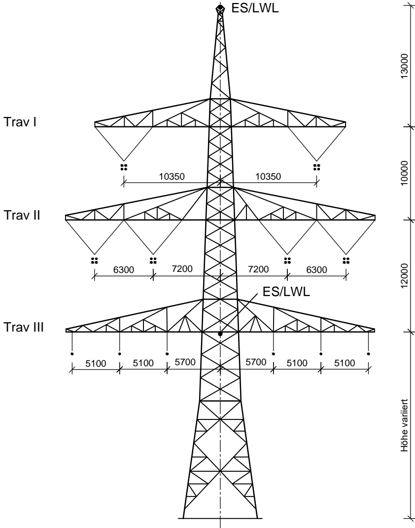
Tragmast T2; DA-4-DE Ltg. Nr. B161: Mast-Nr. 95
