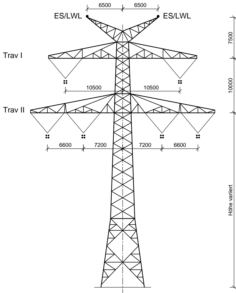
Tragmast T2; D-2-D Ltg. Nr. B161: Mast-Nr. 75
