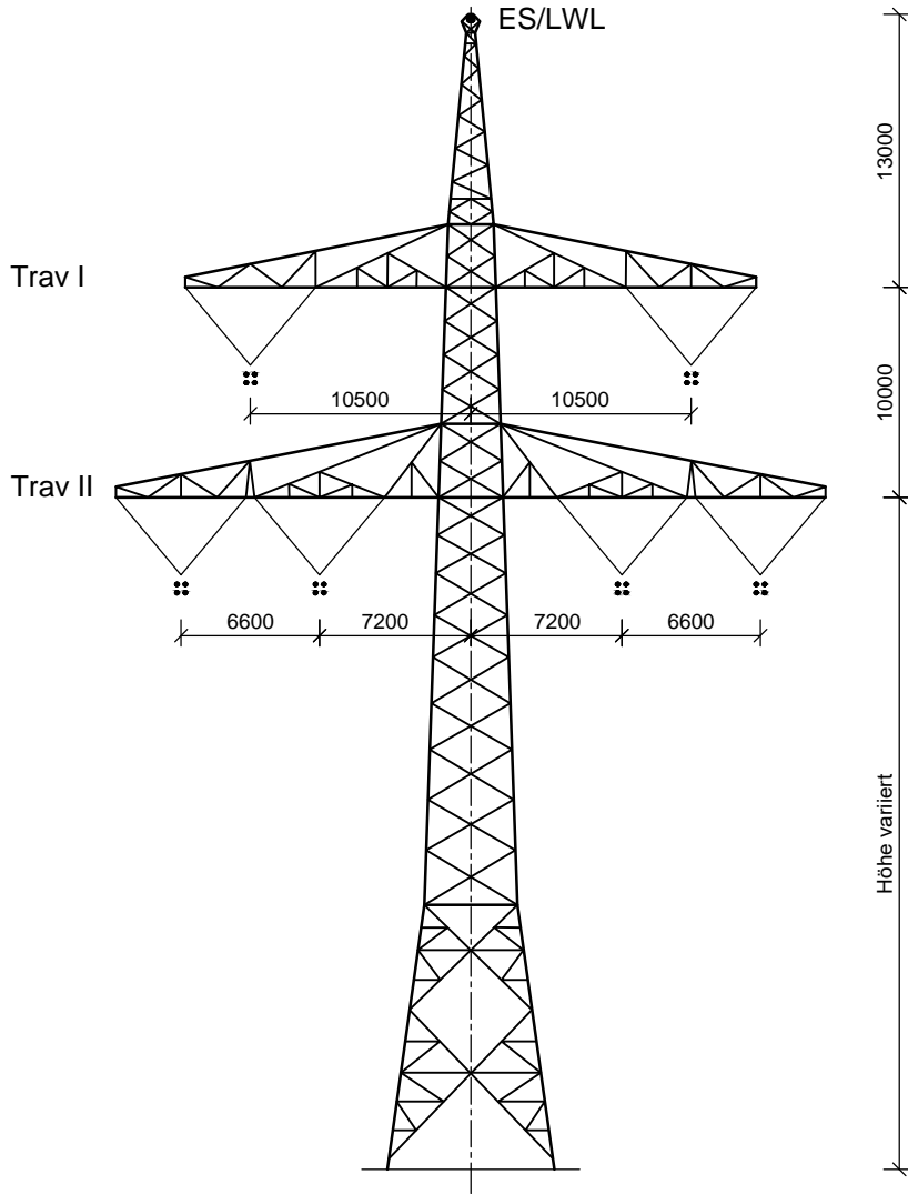
Tragmast T2; D-2-D Ltg. Nr. B161: Mast-Nr. 15, 53, 82, 83, 88
