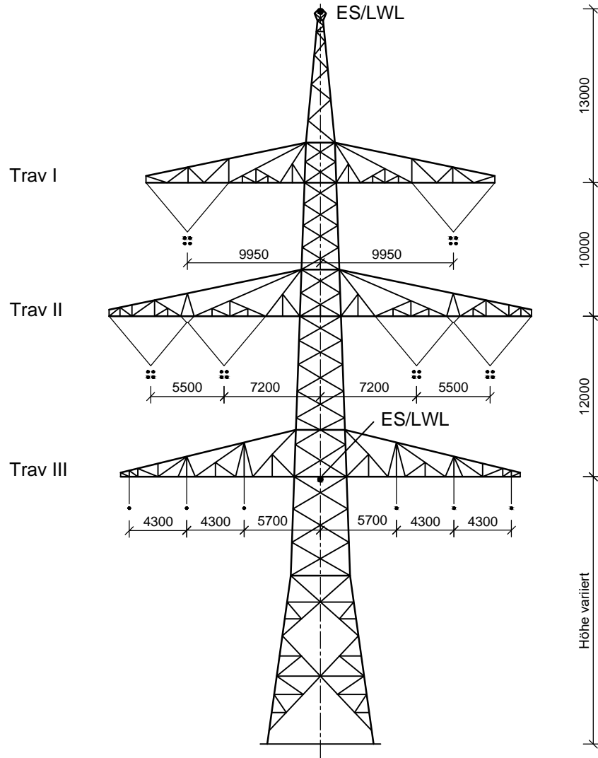
Tragmast T1; DA-4-DE Ltg. Nr. B161: Mast-Nr. 92, 93, 94, 98, 99
