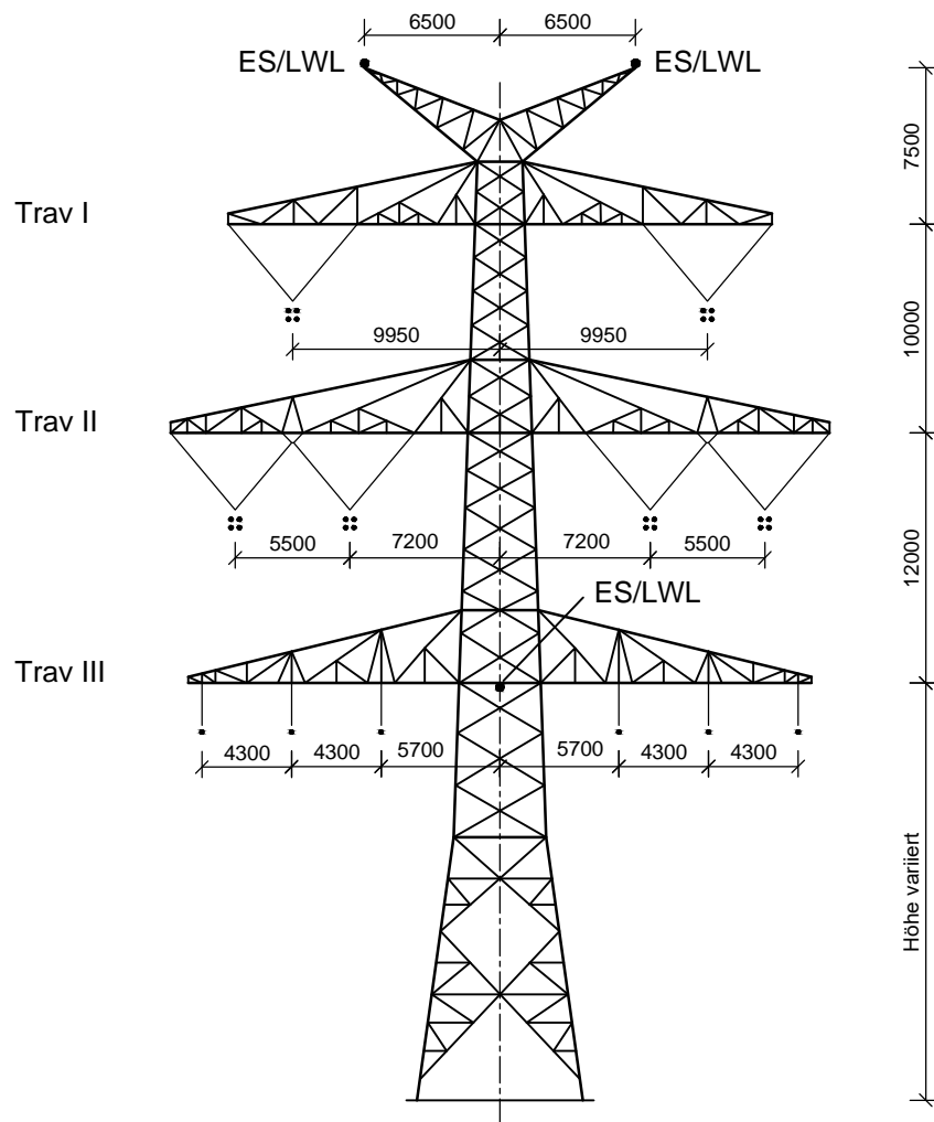
Tragmast T1; DA-4-DE Ltg. Nr. B161: Mast-Nr. 101, 102, 103, 104, 105
