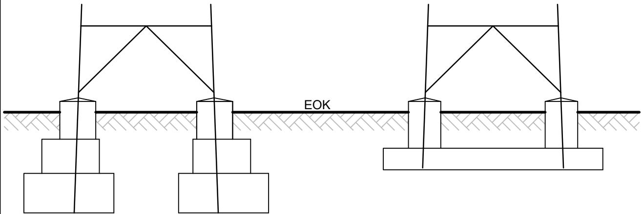
Plattenfundament
