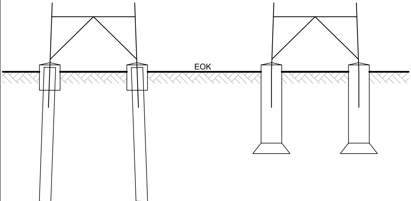
Rammpfahlfundament
