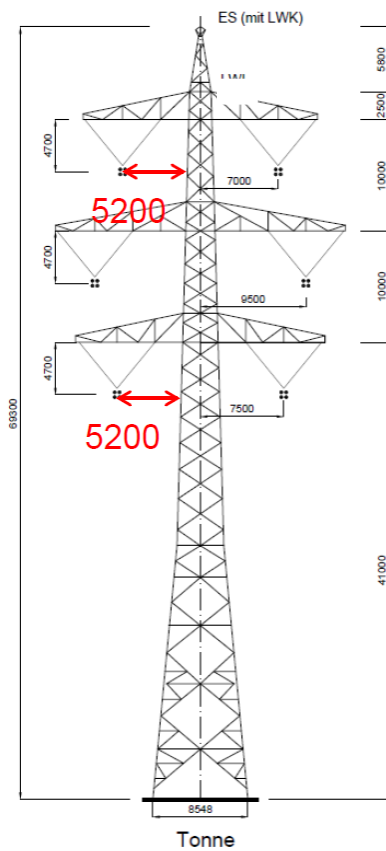
Abbildung 1: Abstand Außenkante Mastschaft zur innersten Phase
