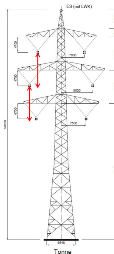
Abbildung 3: Horizontaler Phasenversatz
