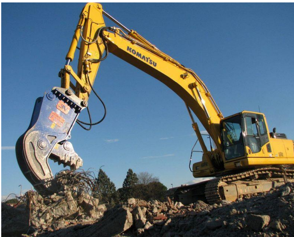
Abbildung 2.2: Bagger mit Abbruchzange (Pulverisierer)
