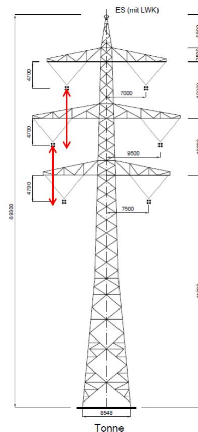
Abbildung 3: Horizontaler Phasenversatz
