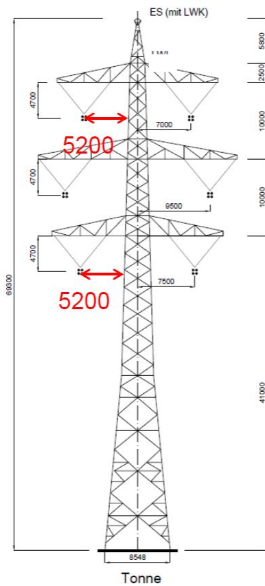
Abbildung 1: Abstand Außenkante Mastchaft zur innersten Phase
