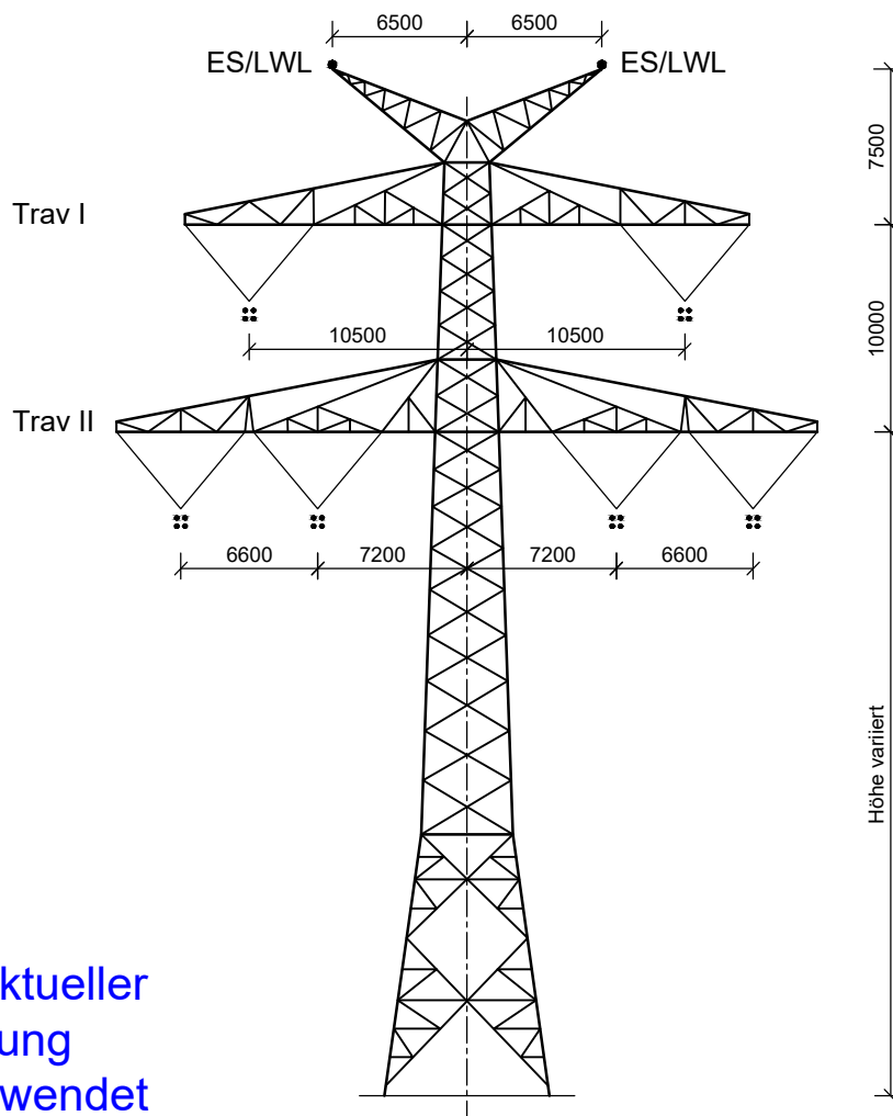
Tragmast T2; D-2-D Ltg. Nr. B161: Mast-Nr. 75
