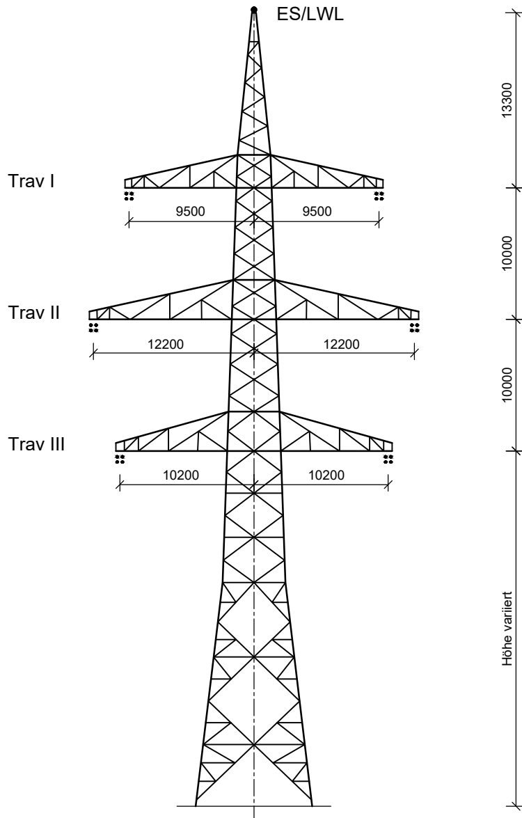
Winkelabspannmast WA120; D-2-T Ltg. Nr. B161: Mast-Nr. 25
