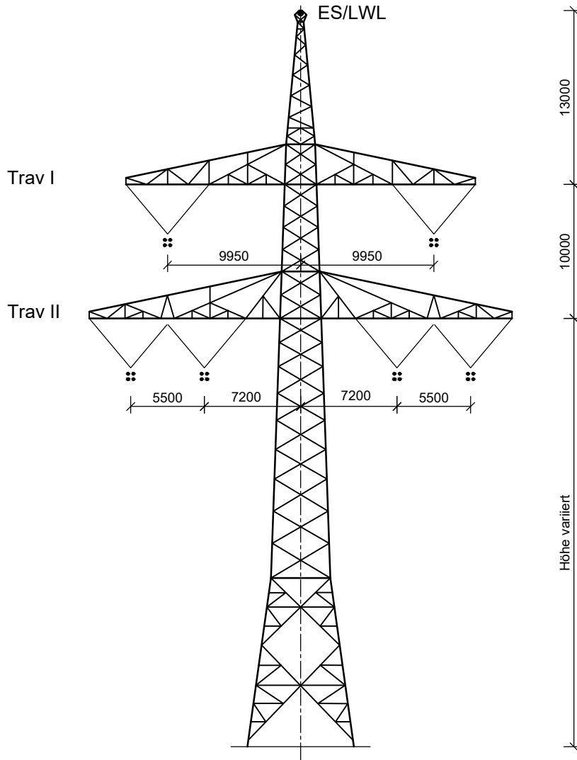
Tragmast T1; D-2-D
