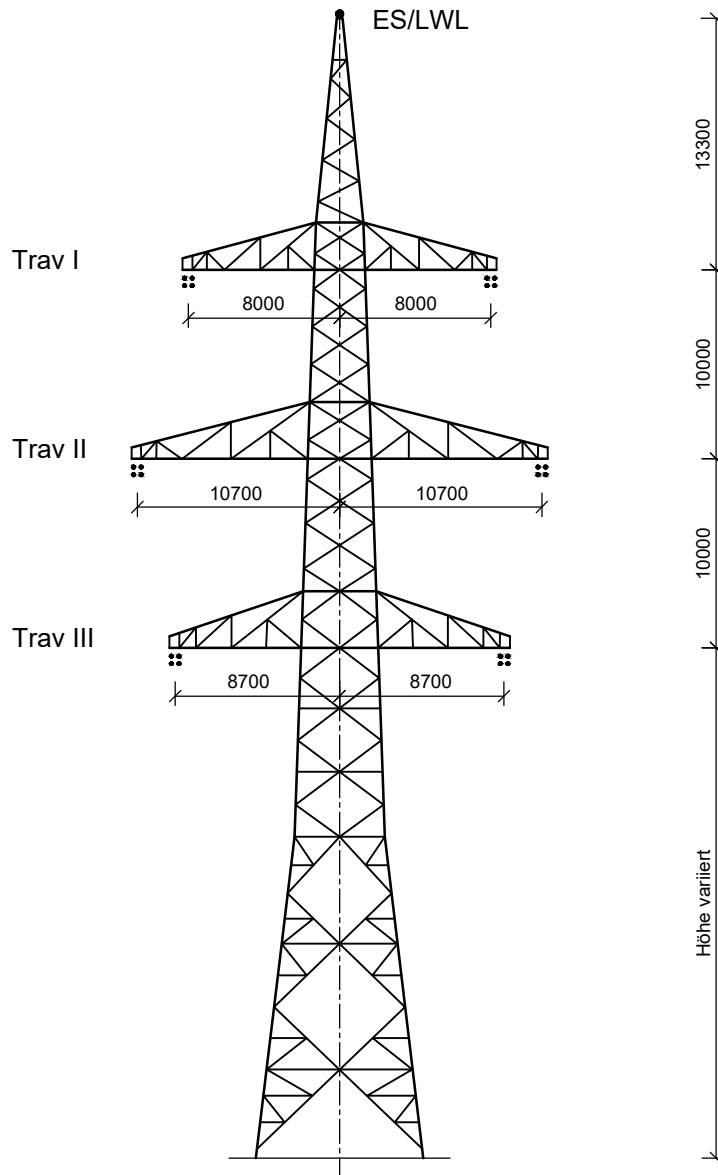
Winkelabspannmast WA140; D-2-T Ltg. Nr. B161: Mast-Nr. 33
