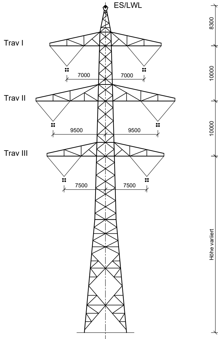
Tragmast T2; D-2-T Ltg. Nr. B161: Mast-Nr. 20
