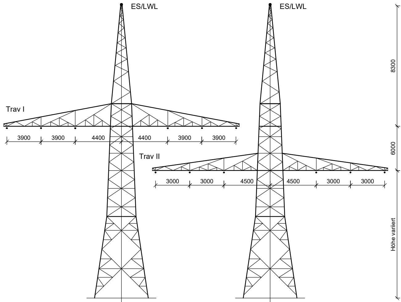
Frontwand - senkrecht zur Leitung
