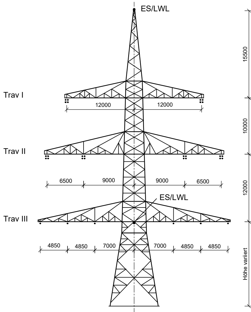
Winkelabspannmast WA140; DA-4-DE Ltg. Nr. B161: Mast-Nr. 100
