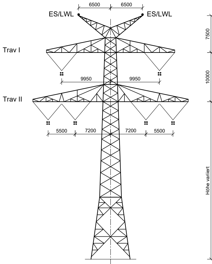
Tragmast T1; D-2-D
