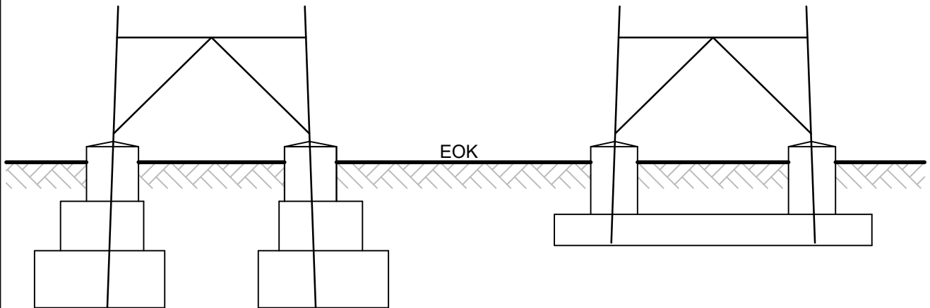
Stufenfundament
